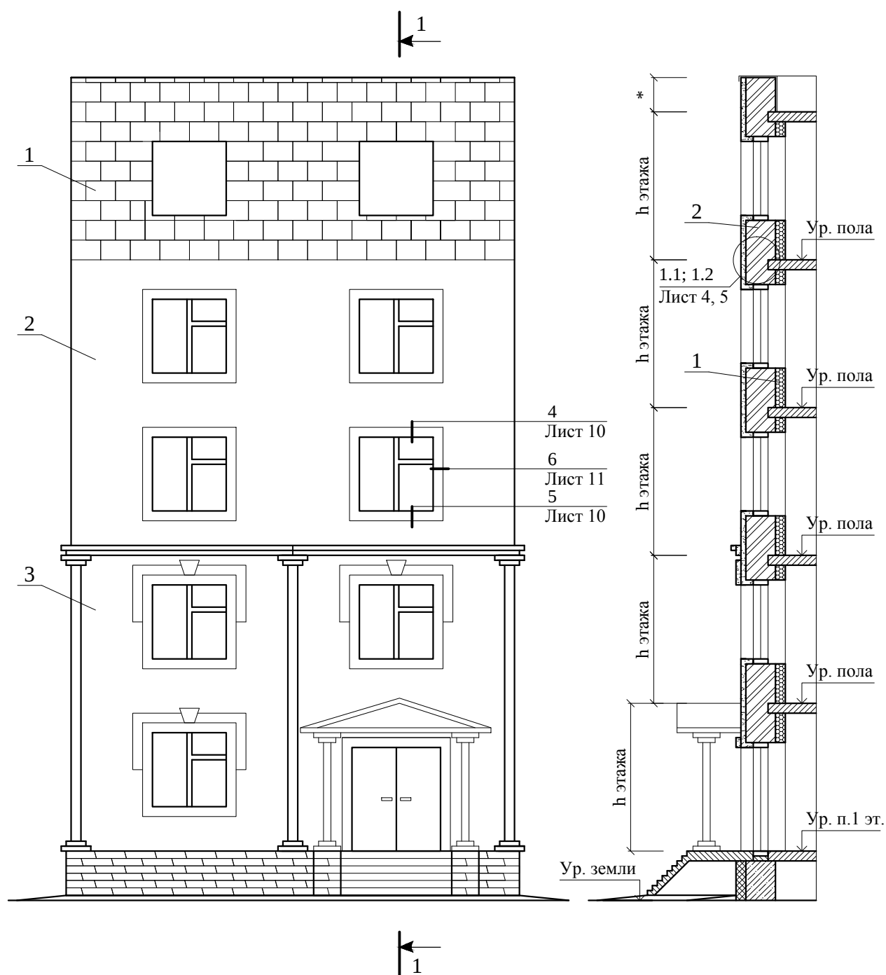
СХЕМА № 1. Расположение плит утеплителя
